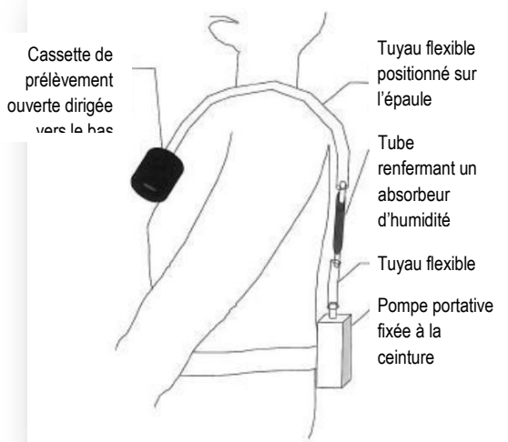
Schéma de la pose d'une pompe sur compagnon
